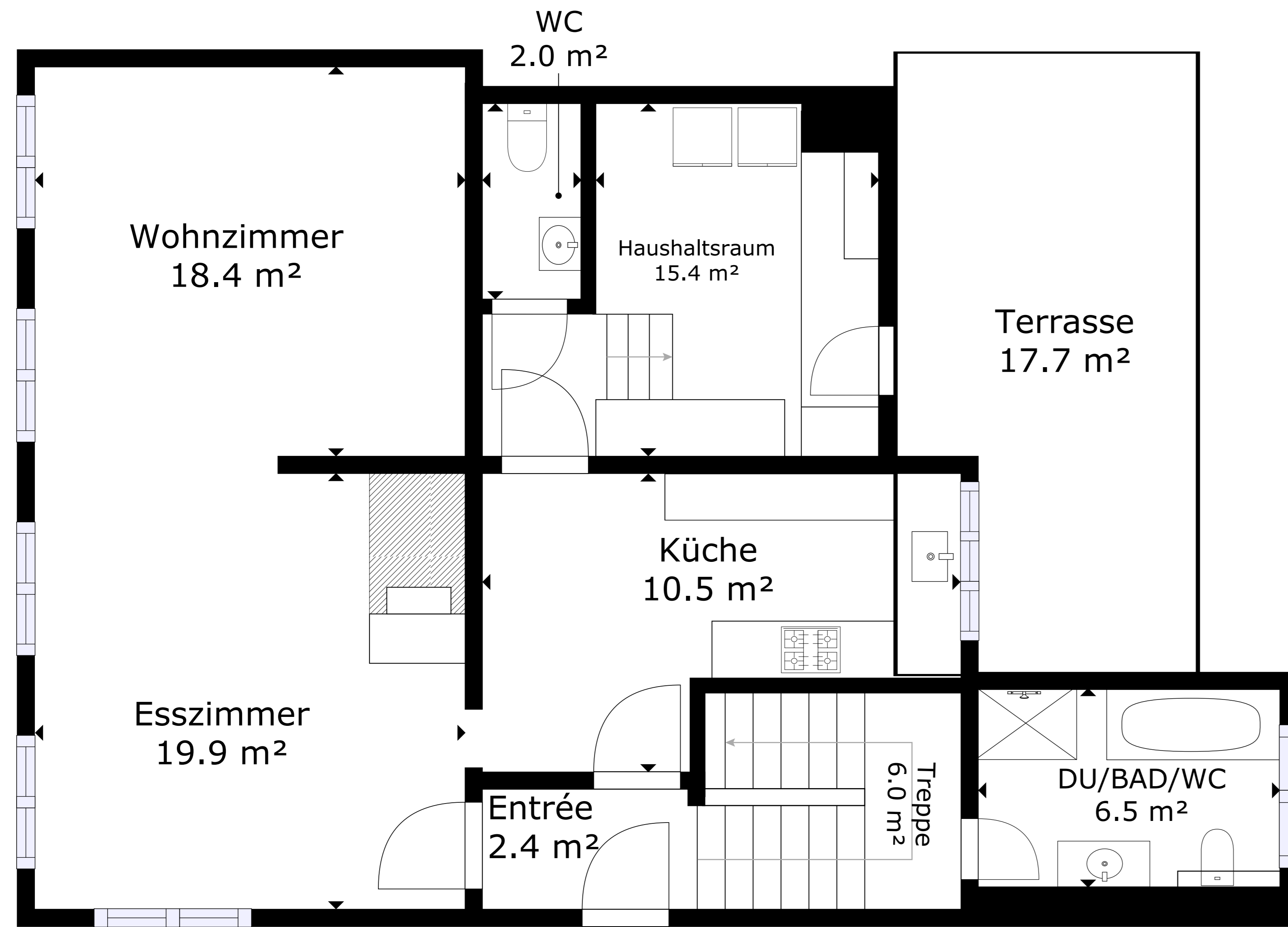
Erdgeschoss 74.6 m 2
